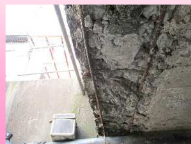
主桁の損傷（鉄筋露出）
