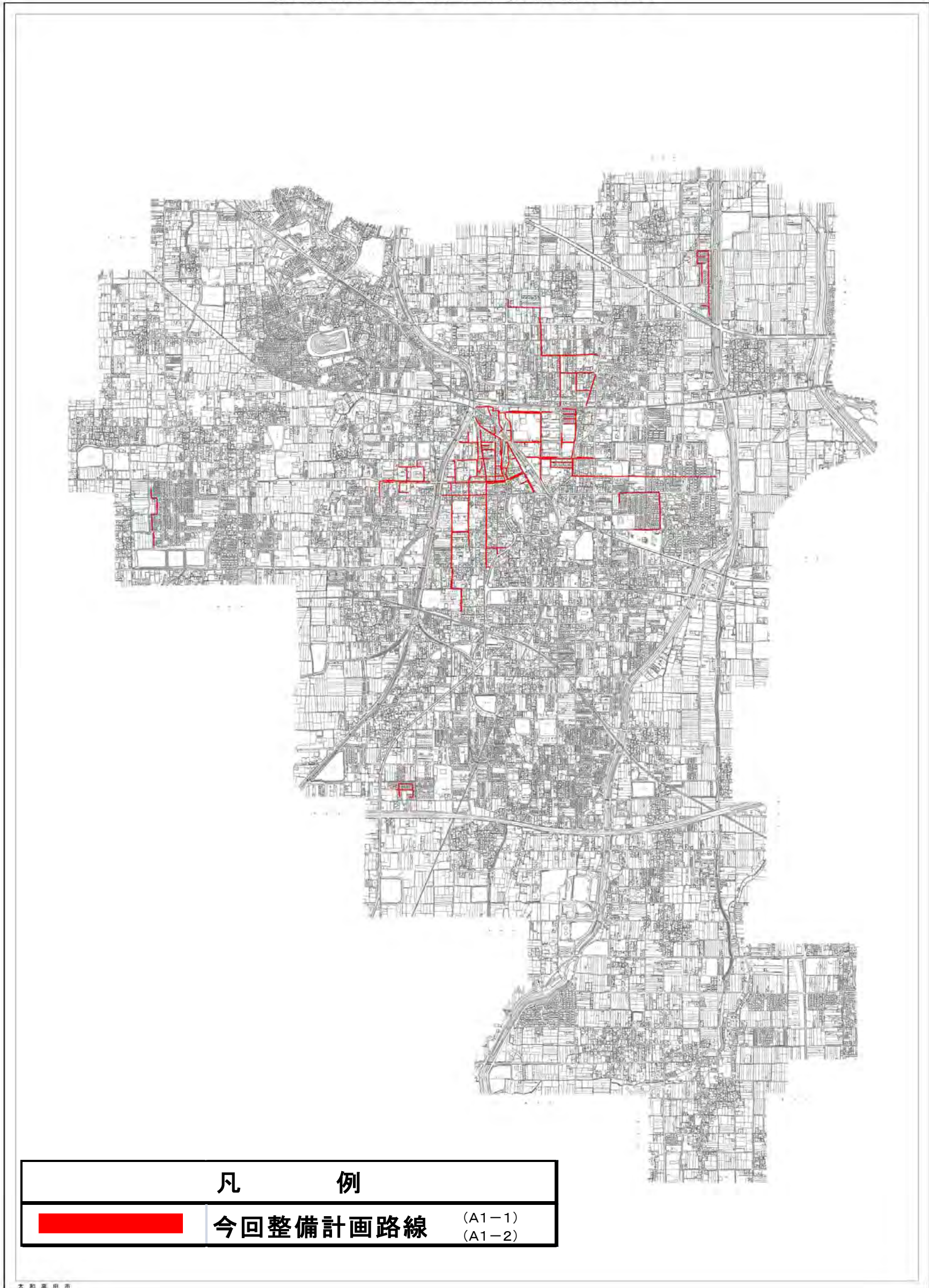
大和高田市公共下水道施設平面図
