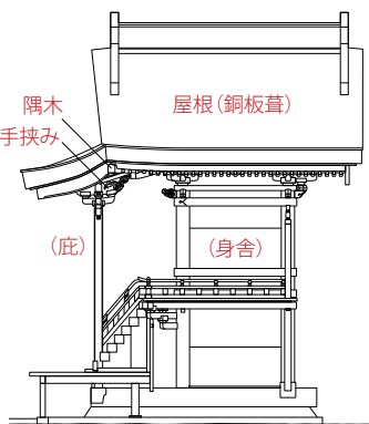
北側面図
