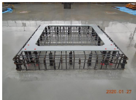
■免震装置下部架台設置状況
