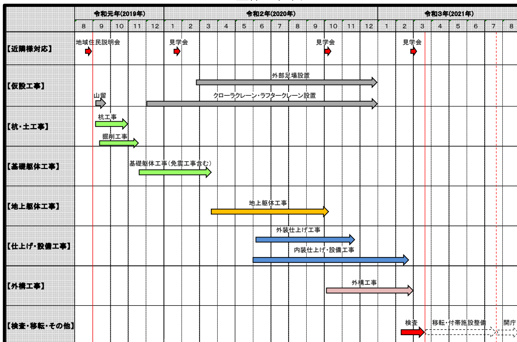
■全体工程表
